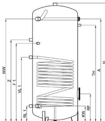
Emaillierter Standspeicher Typ S (mit einem Wärmetauscher)
