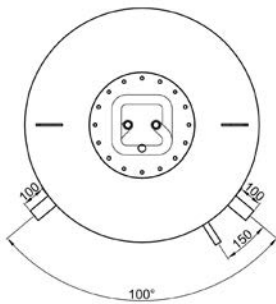
Hygiene-Kombispeicher Typ KE (ohne Wärmetauscher)
