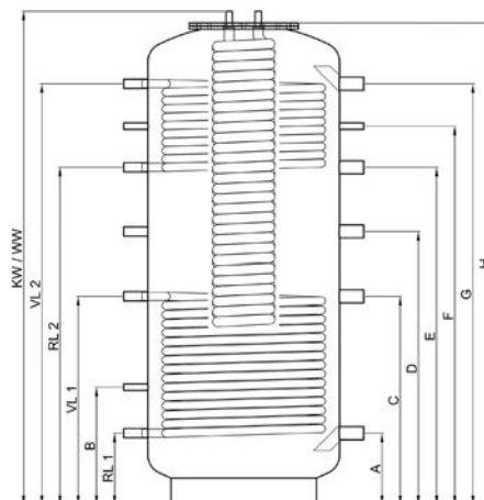
Hygiene-Kombispeicher Typ KER-2 (mit zwei Wärmetauschern)
