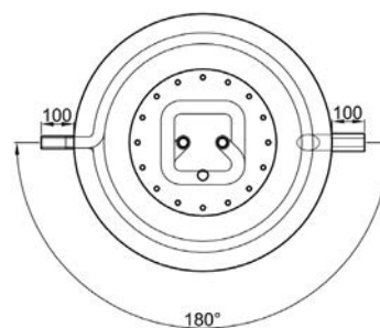
Hygiene-Kombispeicher Typ KER-2 (mit zwei Wärmetauschern)
